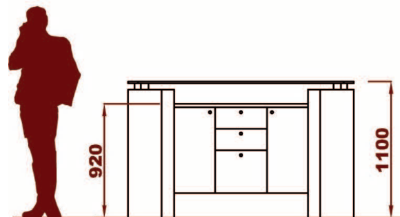
Elévation AA
