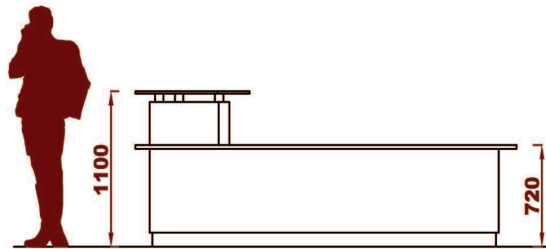
Elévation AA
